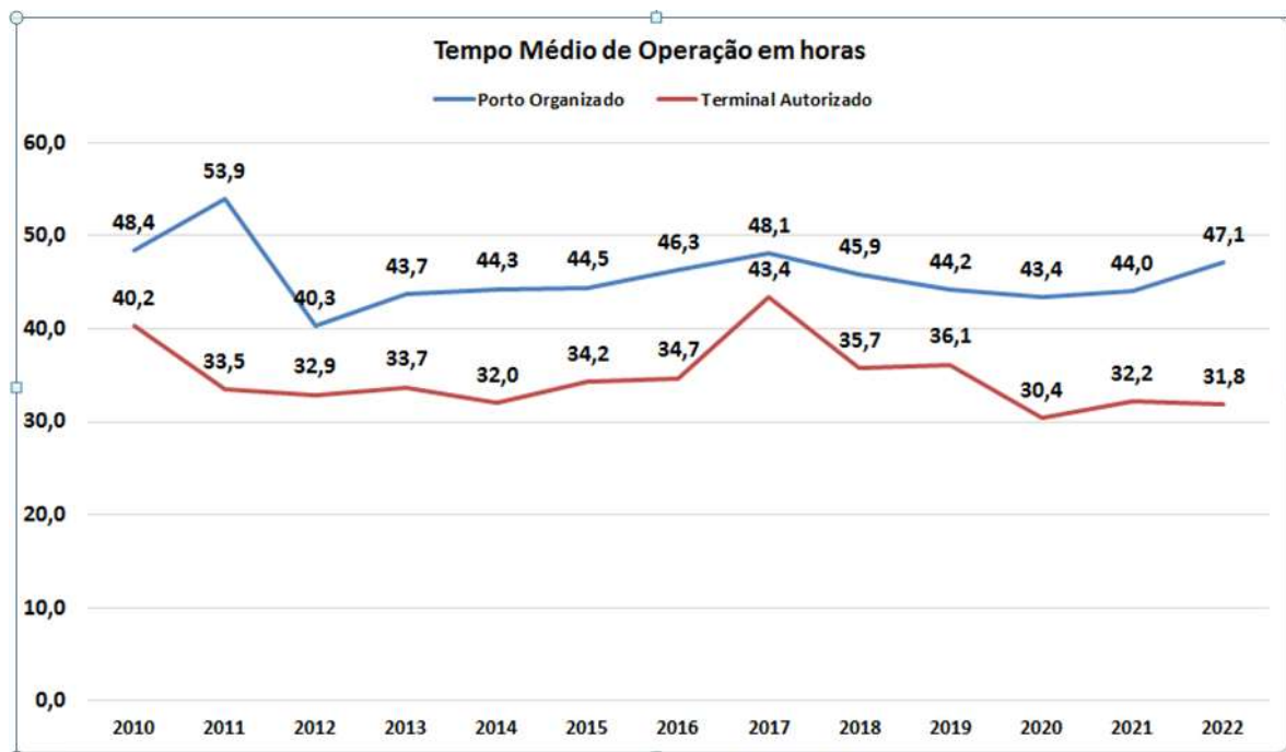
Figura 3 – Gráfico tempo médio de operação./Fonte: autor do artigo, a partir do Painel Estatístico da ANTAQ.
